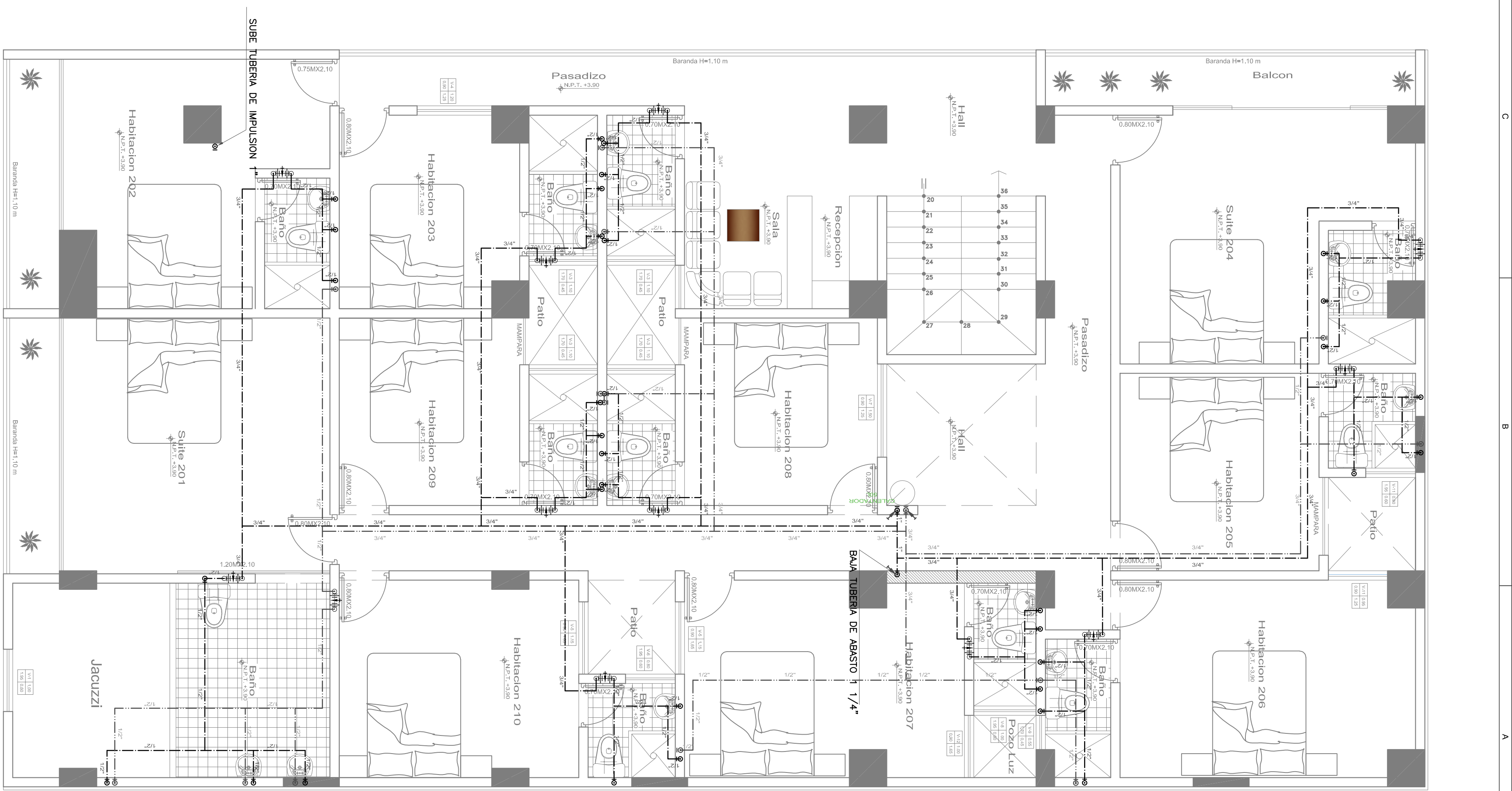
PLANTA: SEGUNDO PISO
