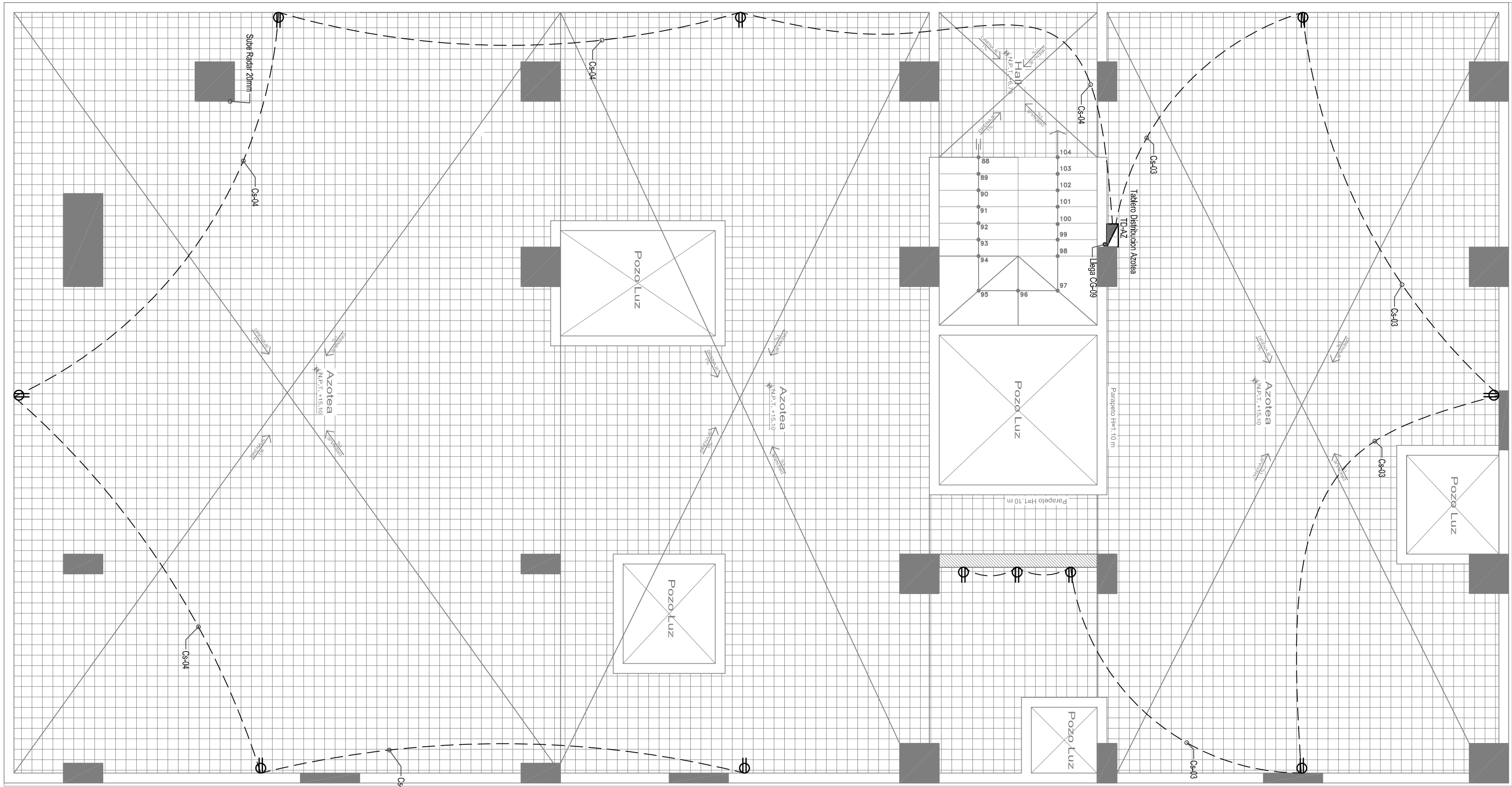
PLANTA: AZOTEA
