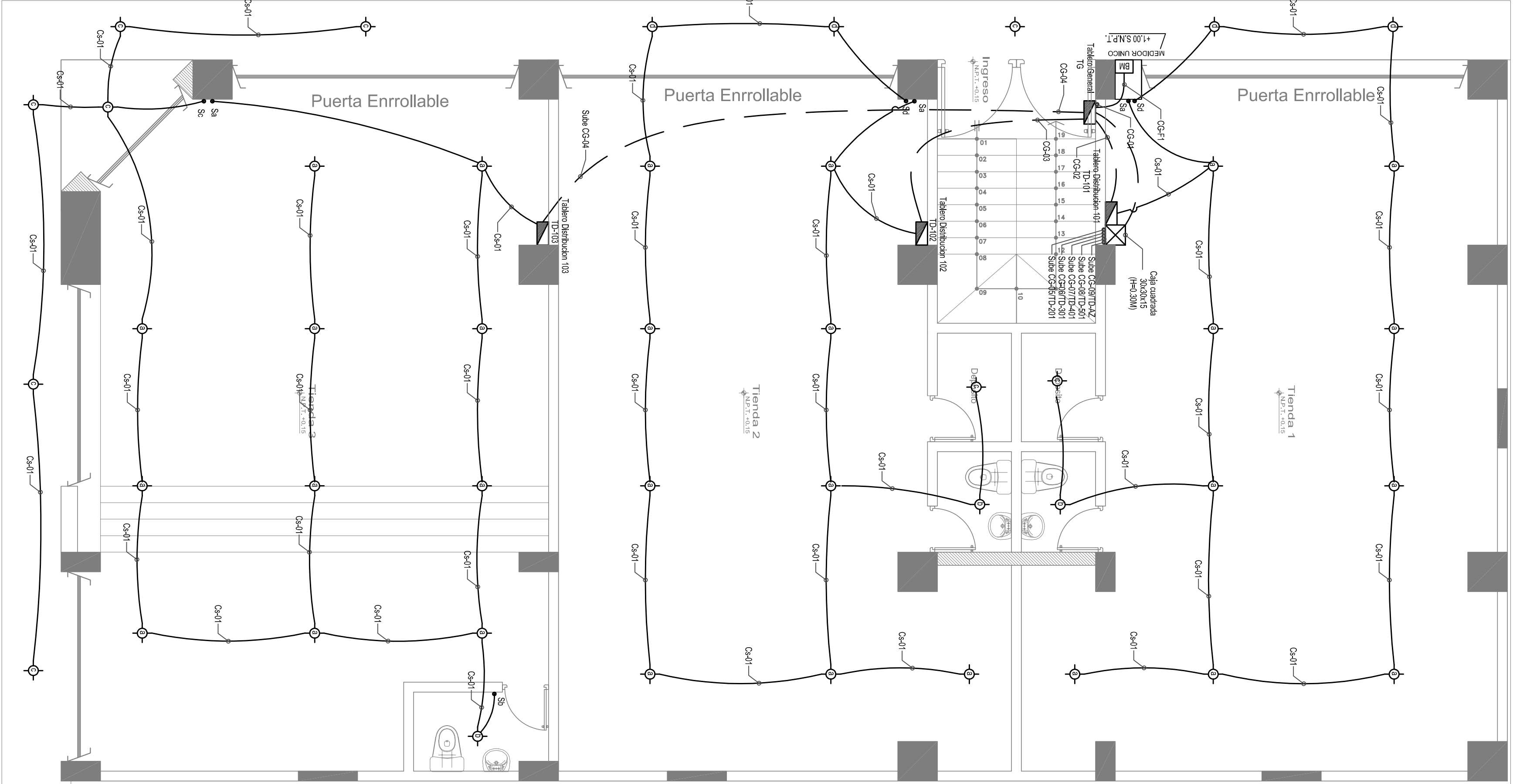
PLANTA: PRIMER PISO ESC.: 1/50
