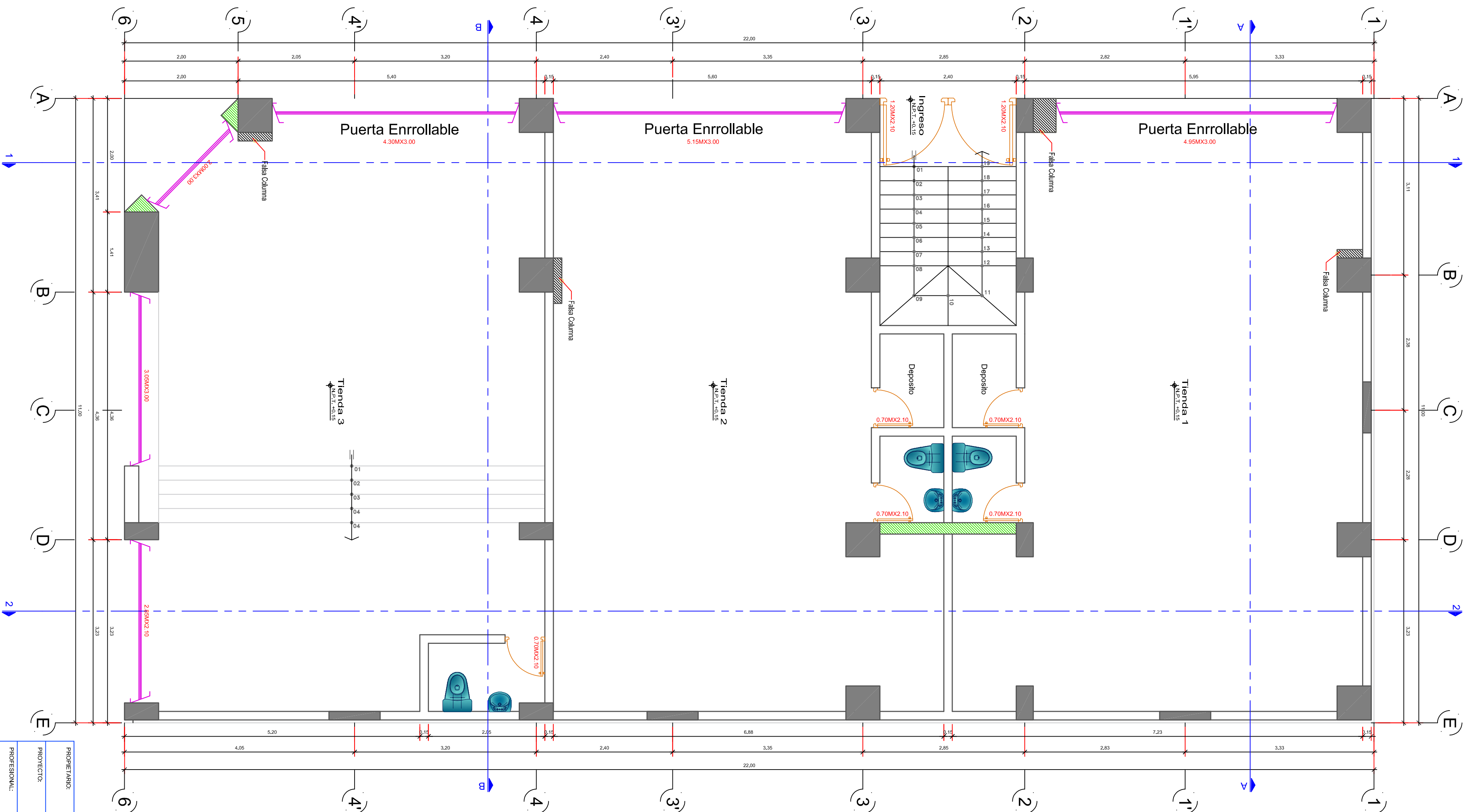
PLANTA: PRIMER PISO
