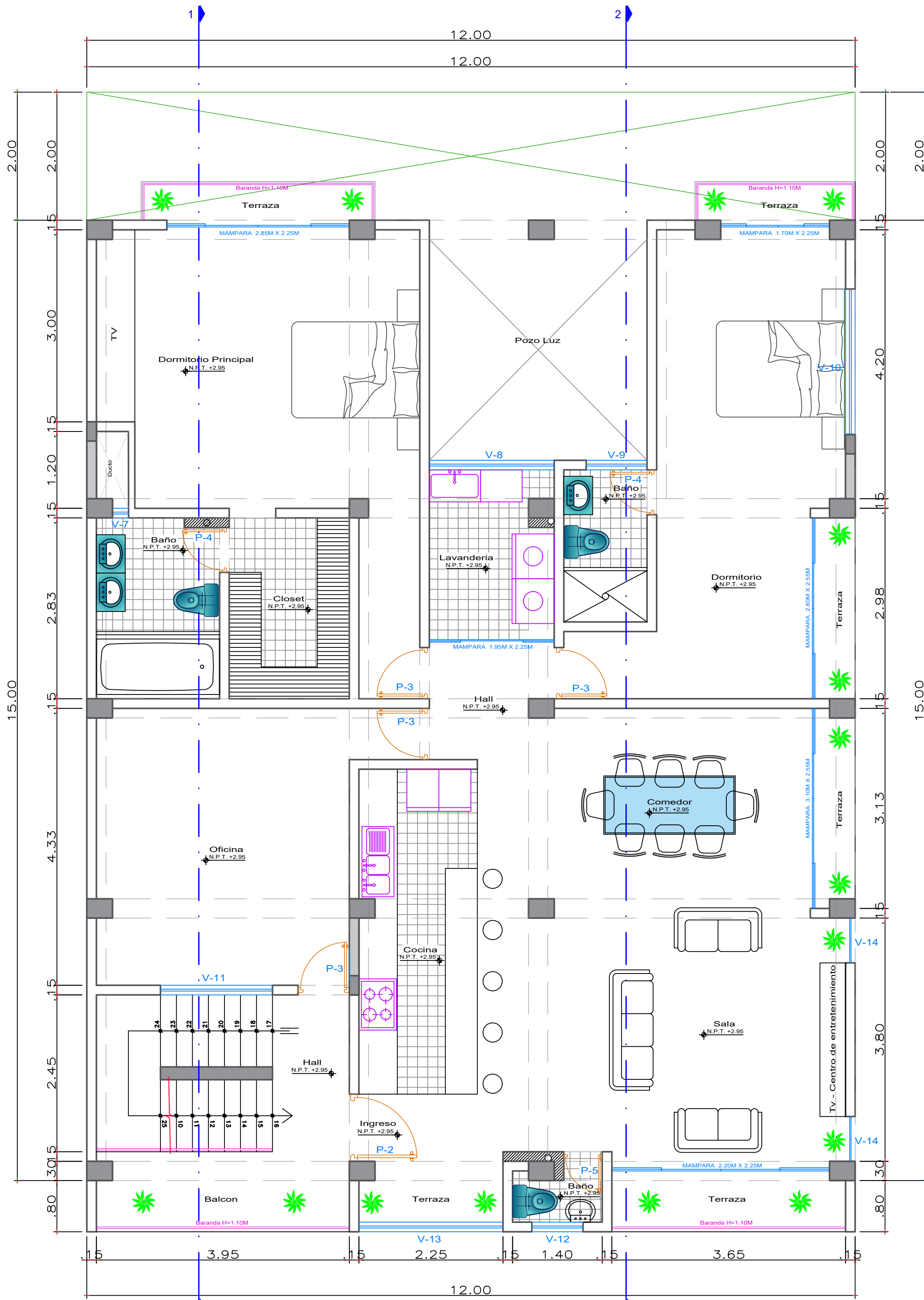
Segundo Piso
