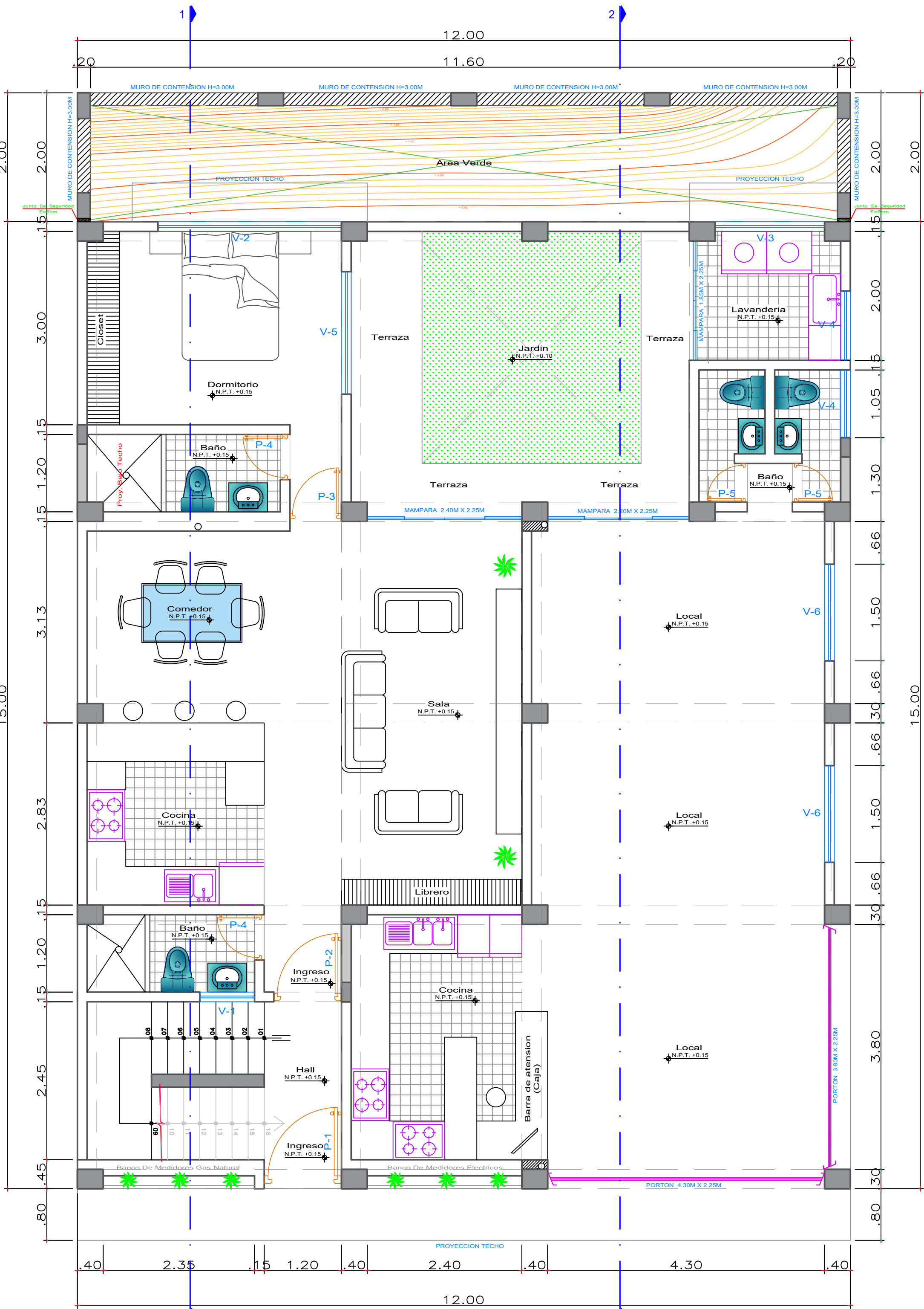
Primer Piso
