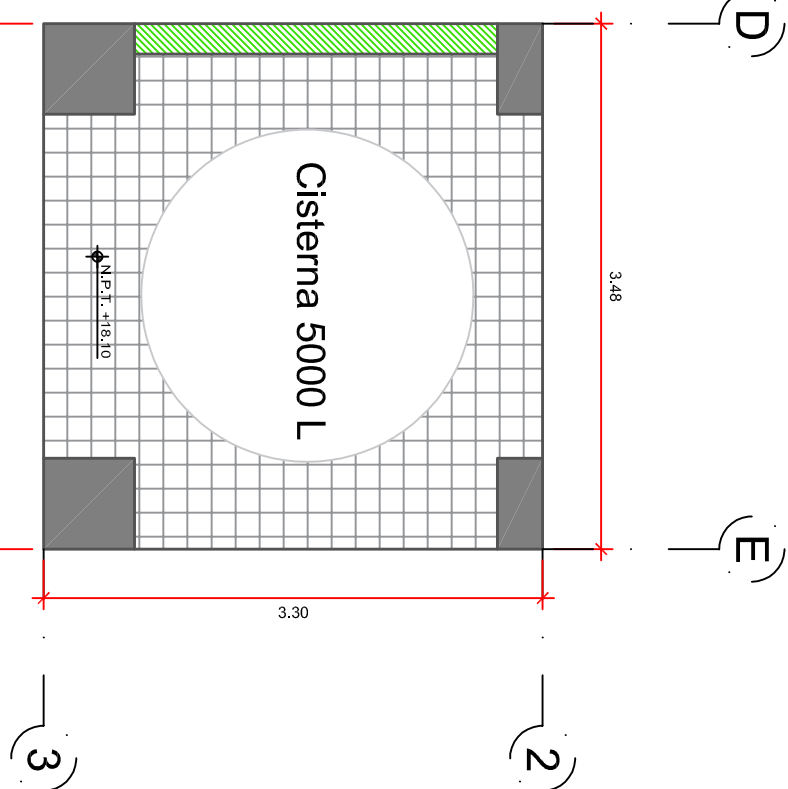
PLANTA: TANQUE
